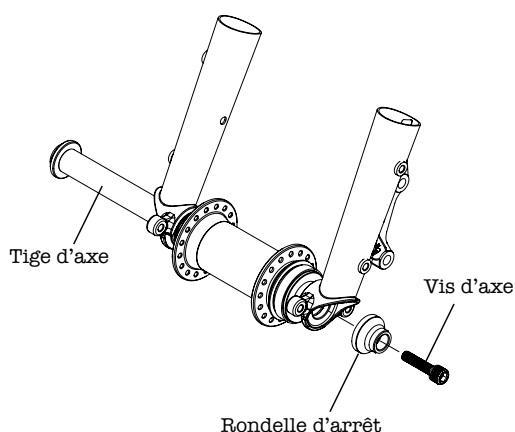
Ensemble d'axe avant
