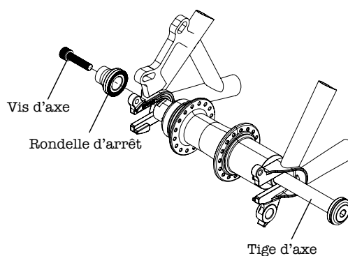
Ensemble d'axe arrière
